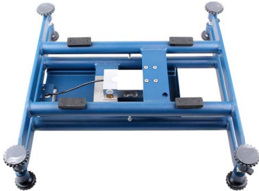
Typical model TN6060-zzzkg sub-frame / Sous-châssis typique du modèle TN6060-zzzkg
